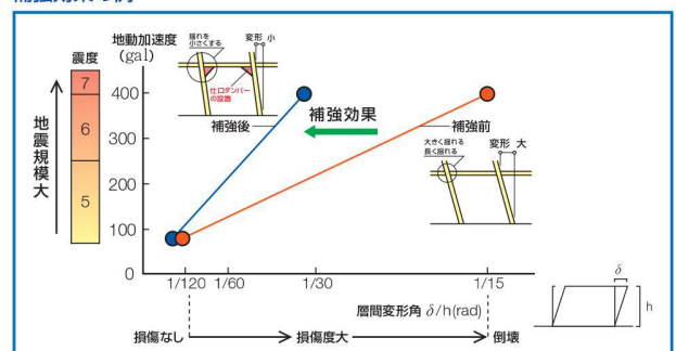
補強効果の例
