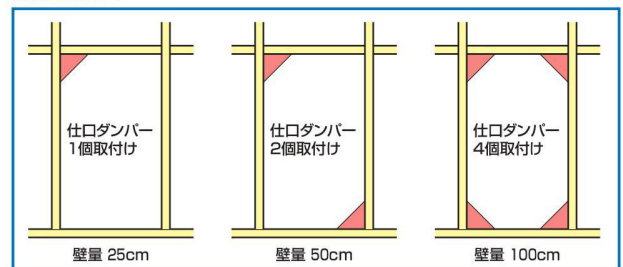
壁倍率換算図
